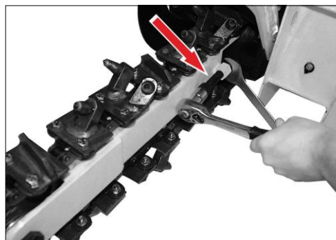
Șurub de reglare a întinderii lanțului
